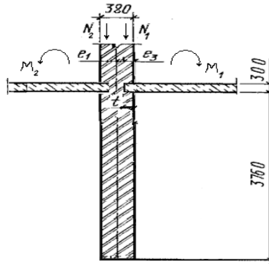
Рисунок 1–Схема простенка
